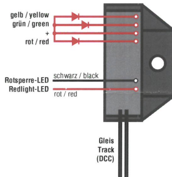
Abbildung 2: Anschlussbelegung Illustration 2: Connection diagram
